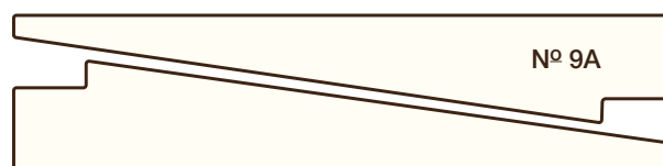
LAMBRIS À DECLIN 6/4; JOINT À MI-BOIS
